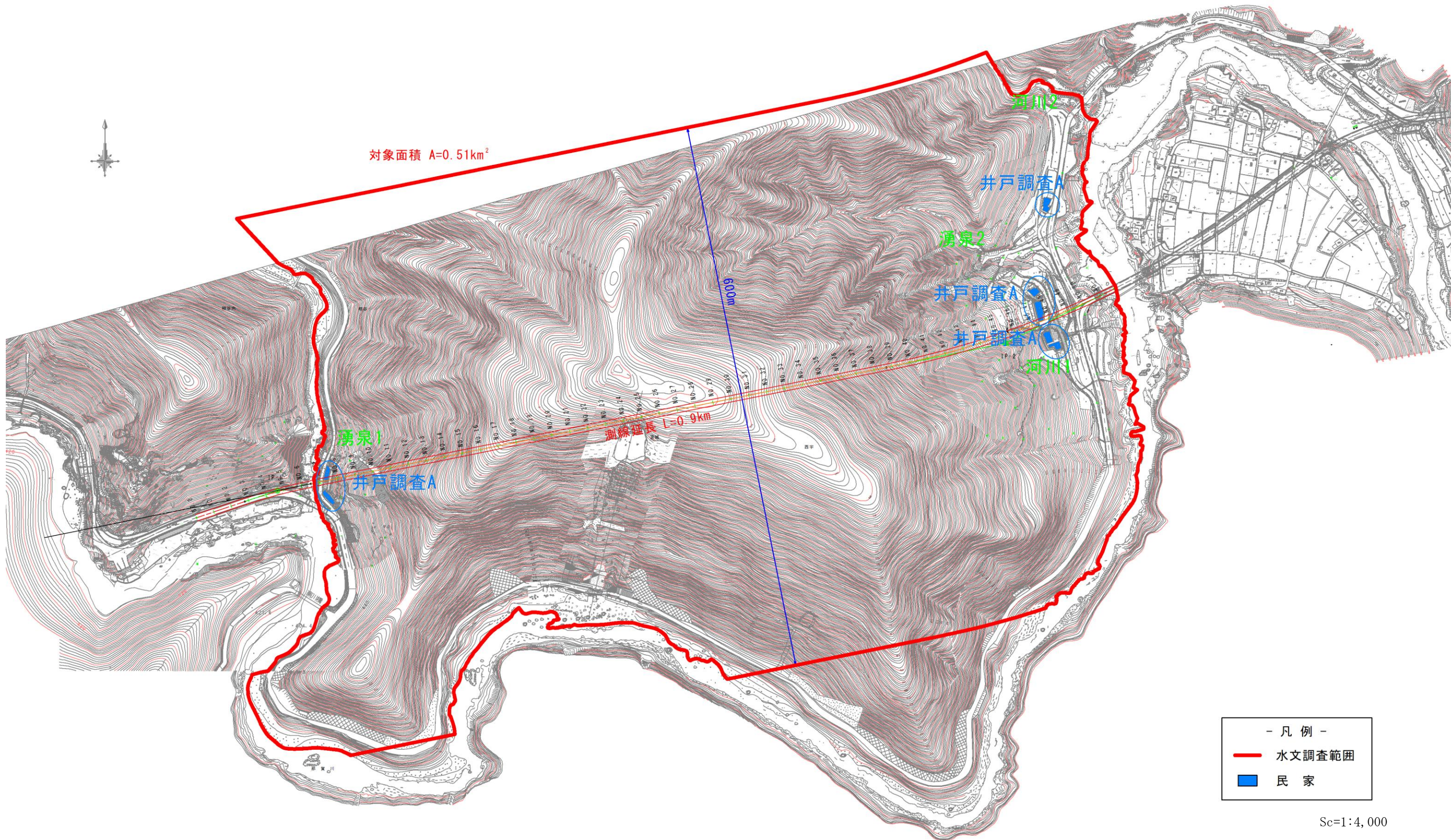
図1 調査計画平面図
